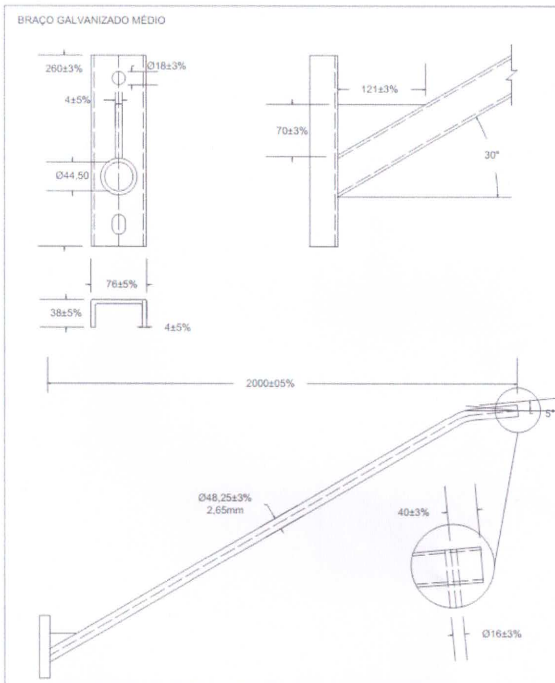
Figura 1 – Braço galvanizado de 2 metros projeção.
