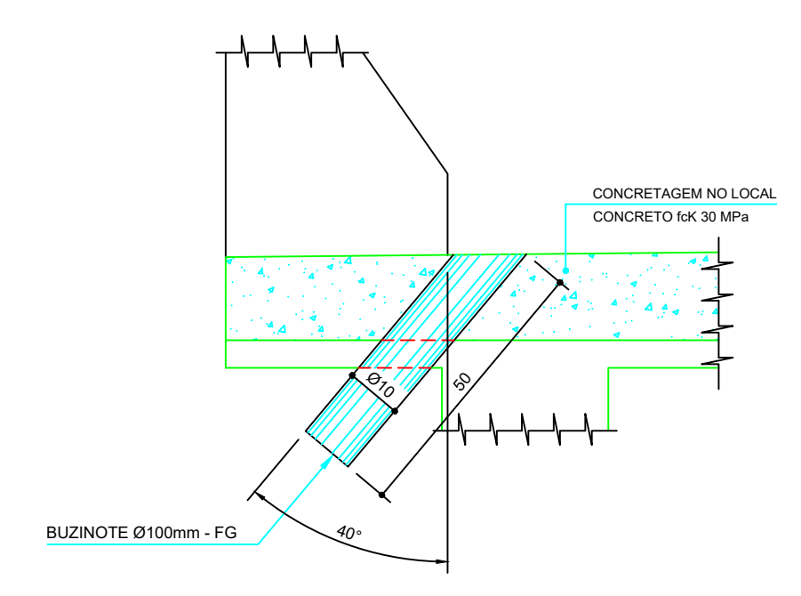
DETALHE DOS BUZINOTES - Ø100mm - (30x) ESC 1:10
