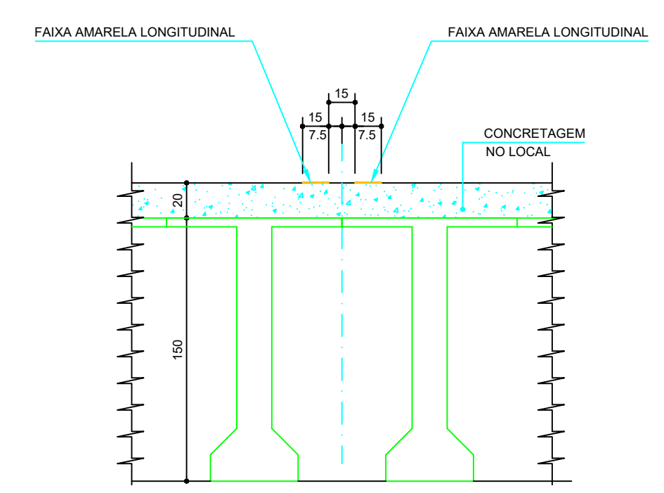
DETALHE A ESC 1:25
