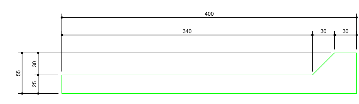
DETALHE DA PLACA DE APROXIMAÇÃO SEÇÃO TRANSVERSAL - FORMA ESC 1:25
