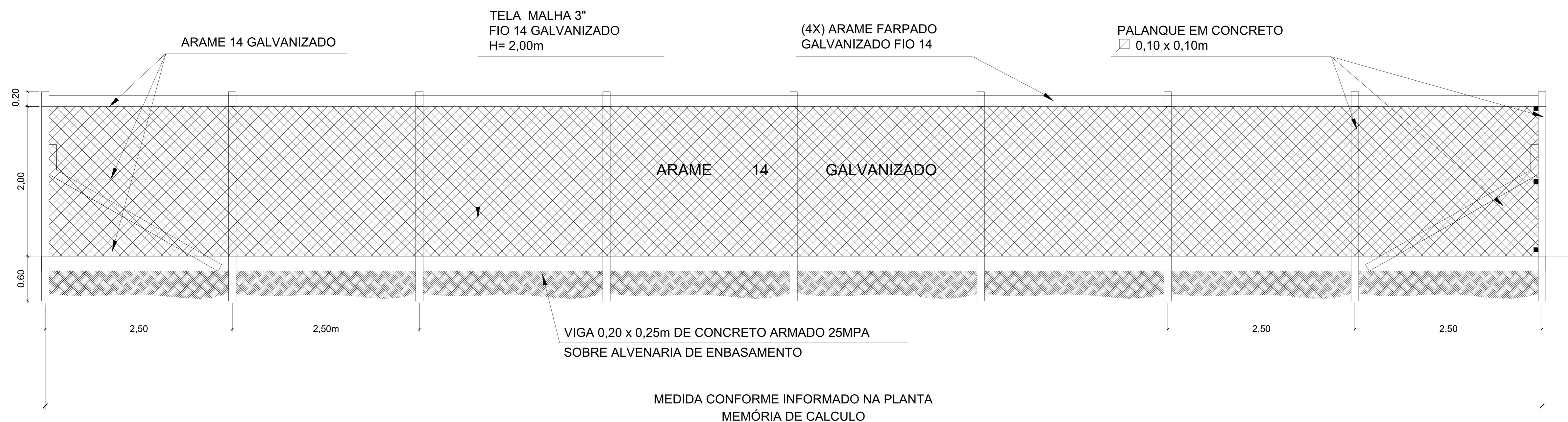
DETALHE "A" - ELEVÇÃO ALAMBRADO ESC 1:25
