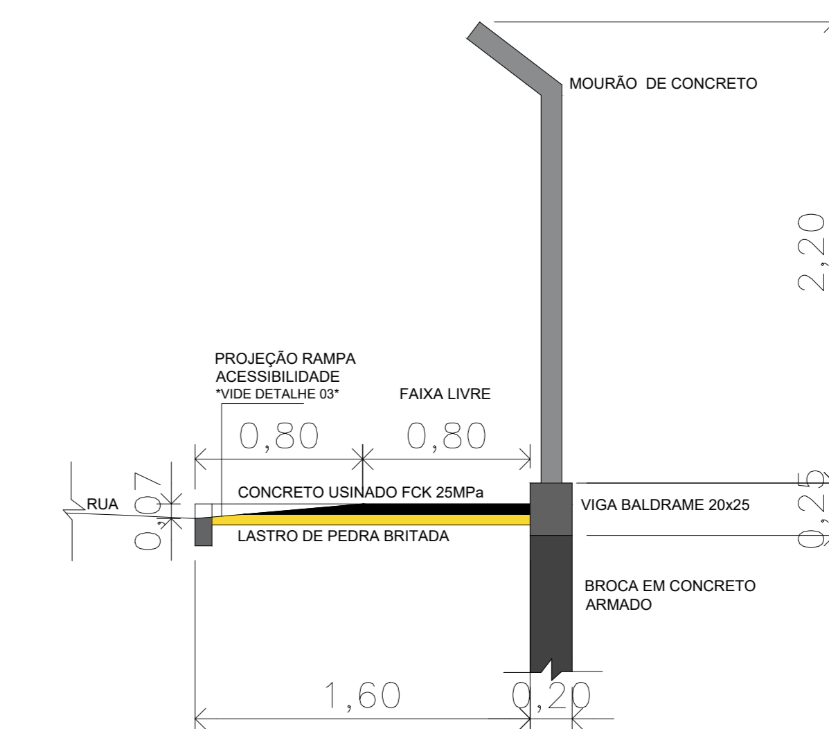
DETALHE 05 ALAMBRADO E CALÇADA ESC: 1/20
