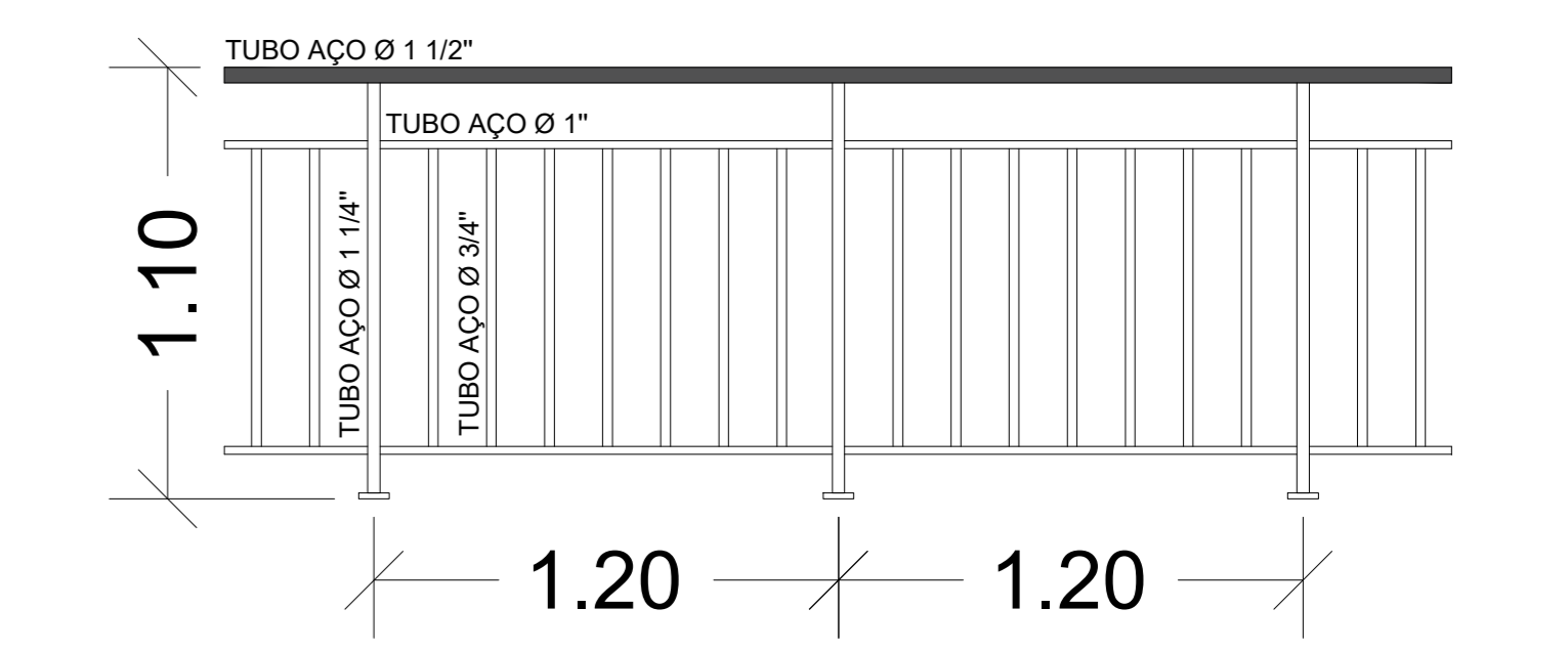
DETALHE 02 GUARDA CORPO ESC: 1/20
