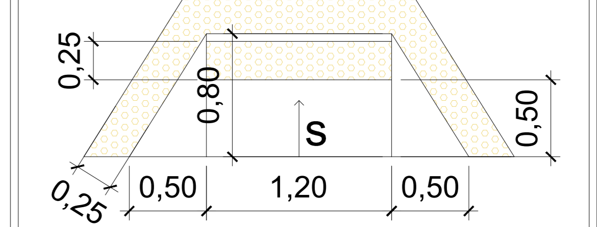
DETALHE 03 RAMPA DE ACESSIBILIDADE ESC: 1/25
