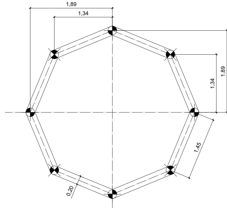
PLANTA FUNDAÇÃO ESC: 1/50
