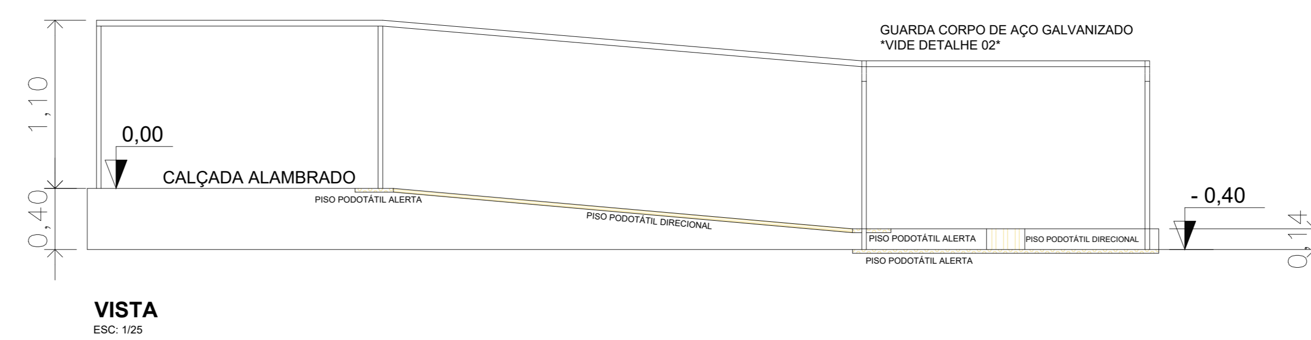
RAMPA ESC: 1/25
