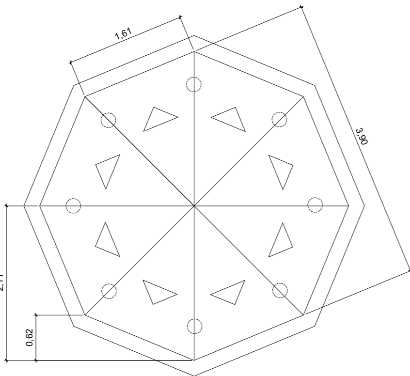
PLANTA COBERTURA ESC: 1/50
