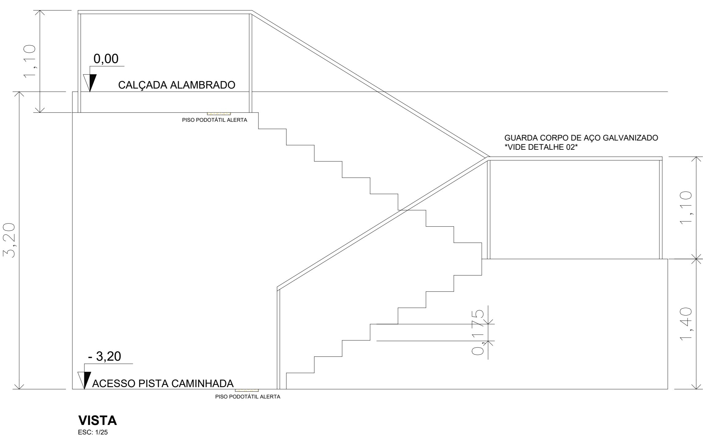
ESCADA ESC: 1/25
