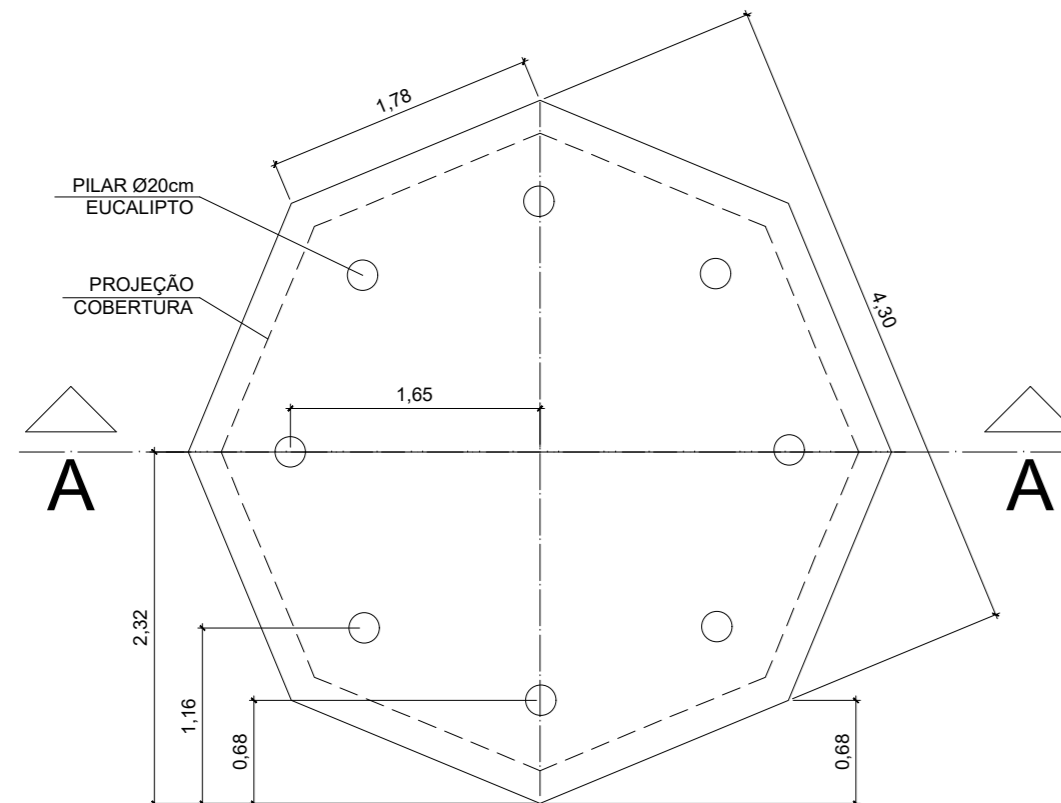
PLANTA BAIXA ESC: 1/50
