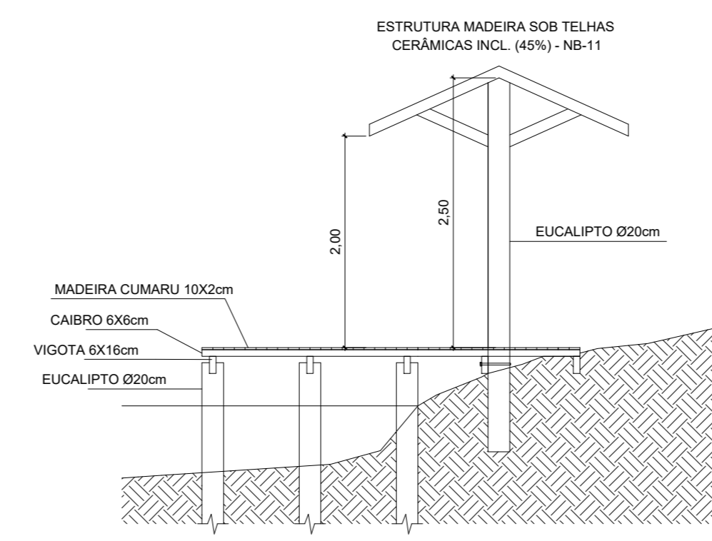
ELEVADO ESC: 1/50
