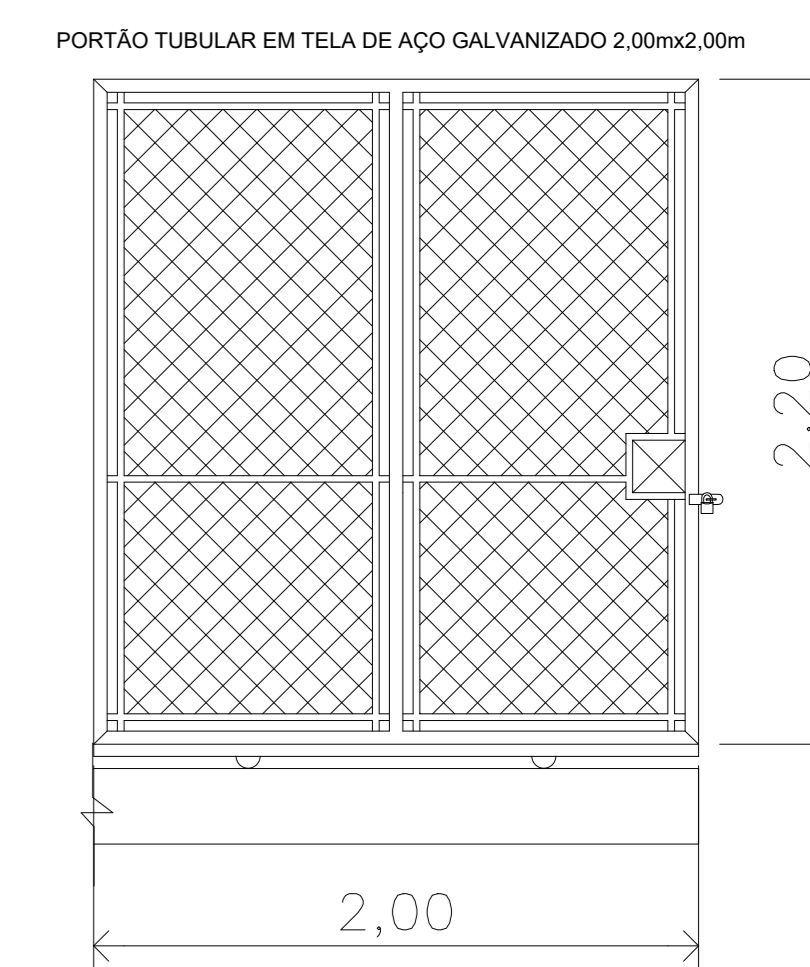
DETALHE 04 PORTÃO TUBULAR ESC: 1/20
