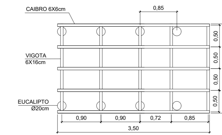
PLANTA ESTRUTURA ESC: 1/50
