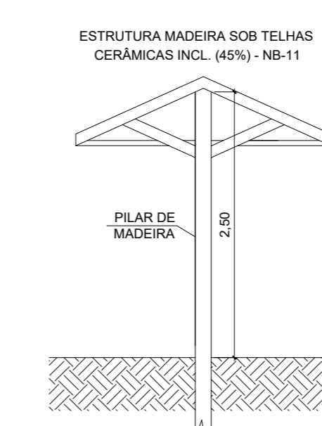
ELEVADO ESC: 1/50
